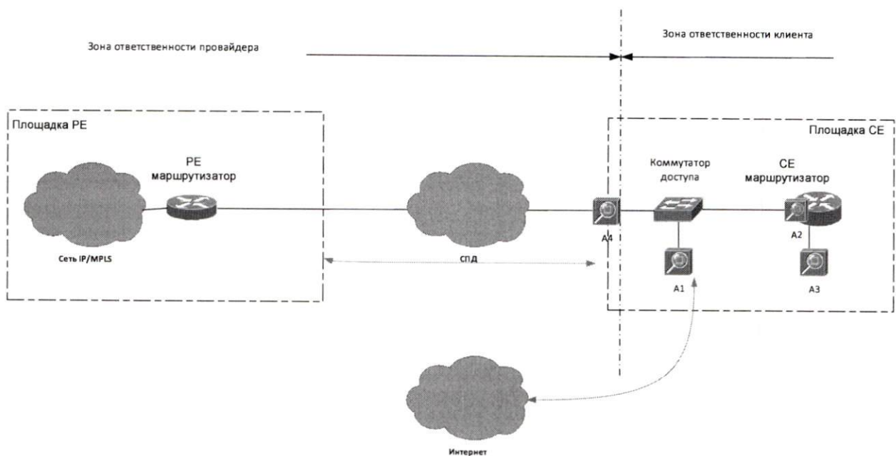
Рис.1. Типовые схемы подключения зондов на площадке типа СЕ
